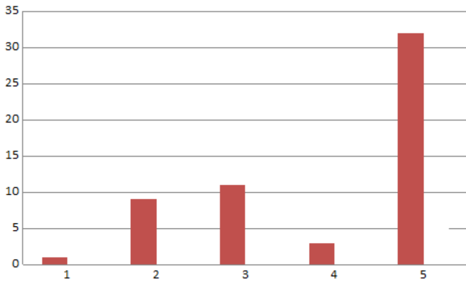
Noten der Modulprüfungen für Grundlagen und Ausbau 1 (SoSe 2015 und WiSe 2015/16)
